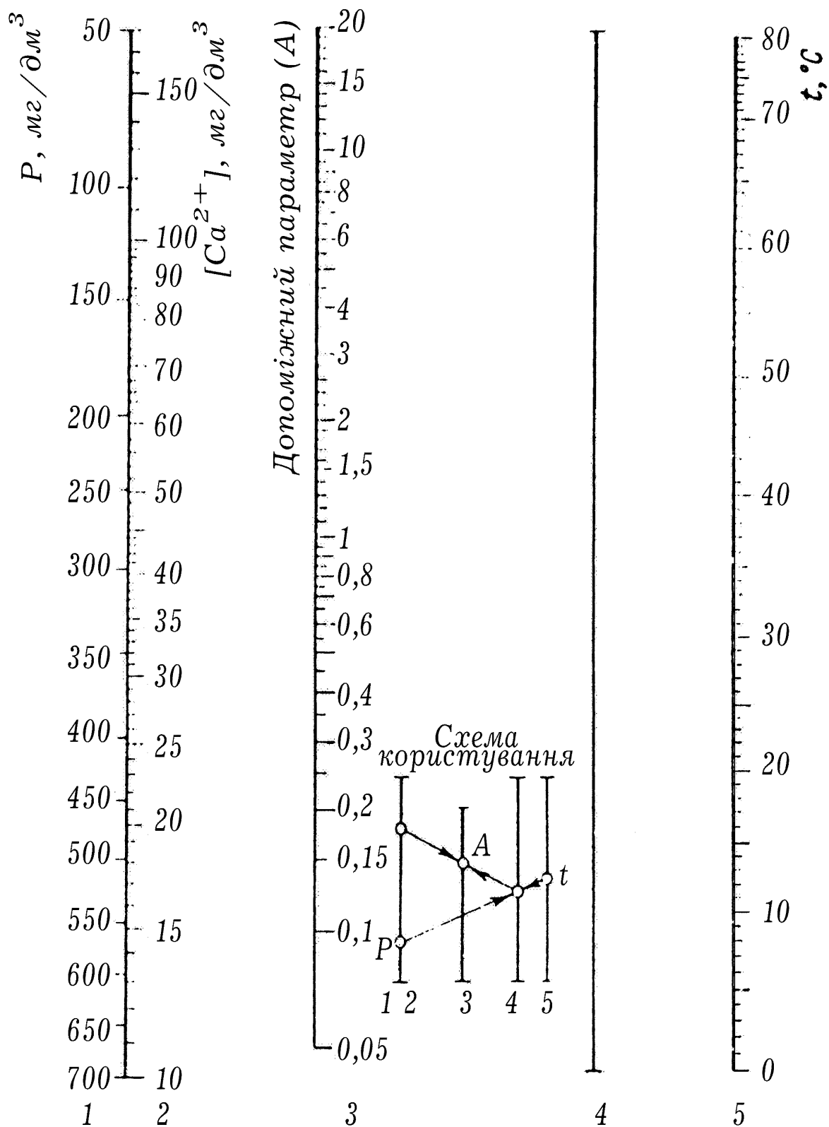
Рис. 2. Номограма визначення допоміжного фактора для розрахування концентрації агресивного оксиду вуглецю (IV) у воді
