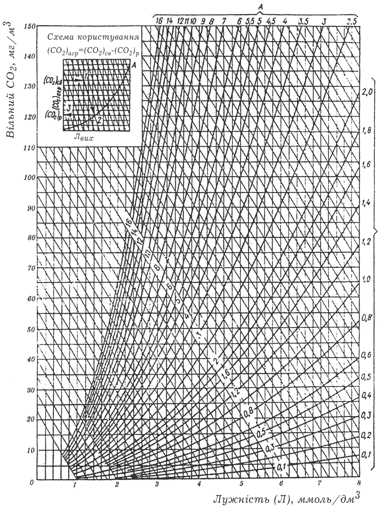
Рис. 3. Номограма визначення концентрації агресивного оксиду вуглецю (IV) у воді
