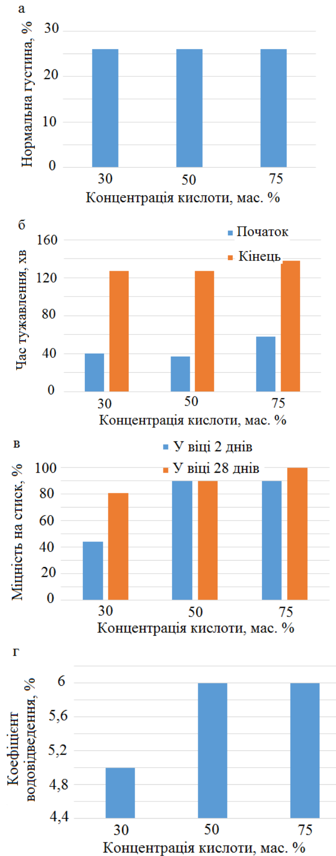
Рис. 2. Властивості цементу, що містить 1,5% шкаралуп волоського горіха модифікованих розчином H_3PO_4 різної концентрації: а – нормальна густина; б – час тужавлення; в – міцність на стиск; г – коефіцієнт водовідведення
