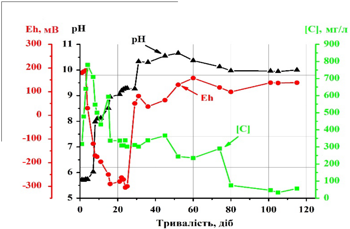
Рис.1. Аеробне очищення токсичного фільтрату після ферментації багатокомпонентних твердих харчових відходів у аеробній пілотній модульній установці
