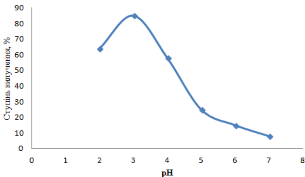
Рис. 2. Вплив рН на ефективність вилучення нафтопродуктів
